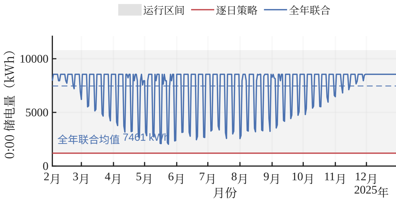
逐日策略与全年联合基准的储电量轨迹
